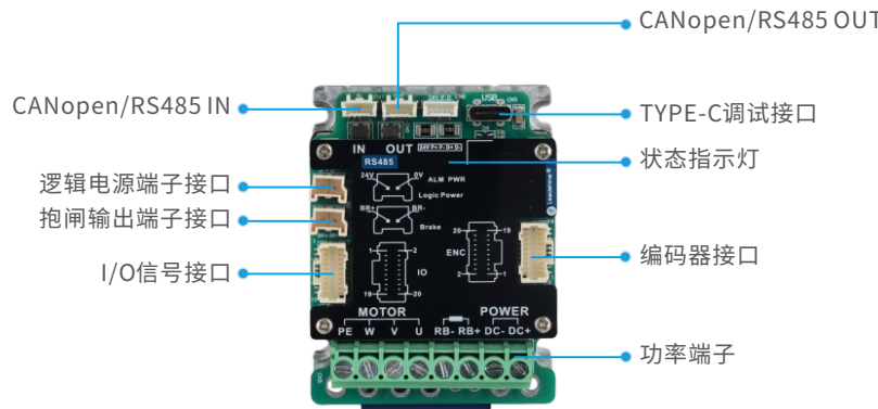
(LD3M-CAN/RS驱动器接口说明)
