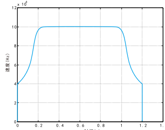
对称S型速度曲线(初末速度可设)
