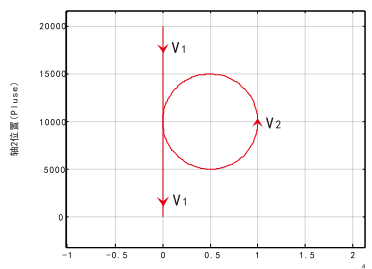
多段连续插补轨迹
