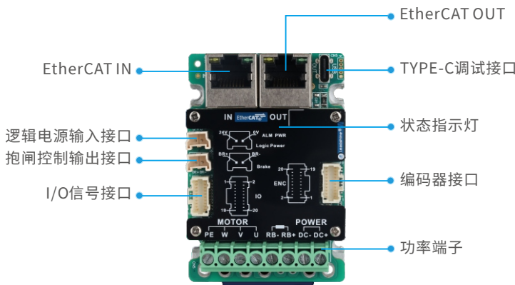
(LD3M-EC驱动器接口说明)
